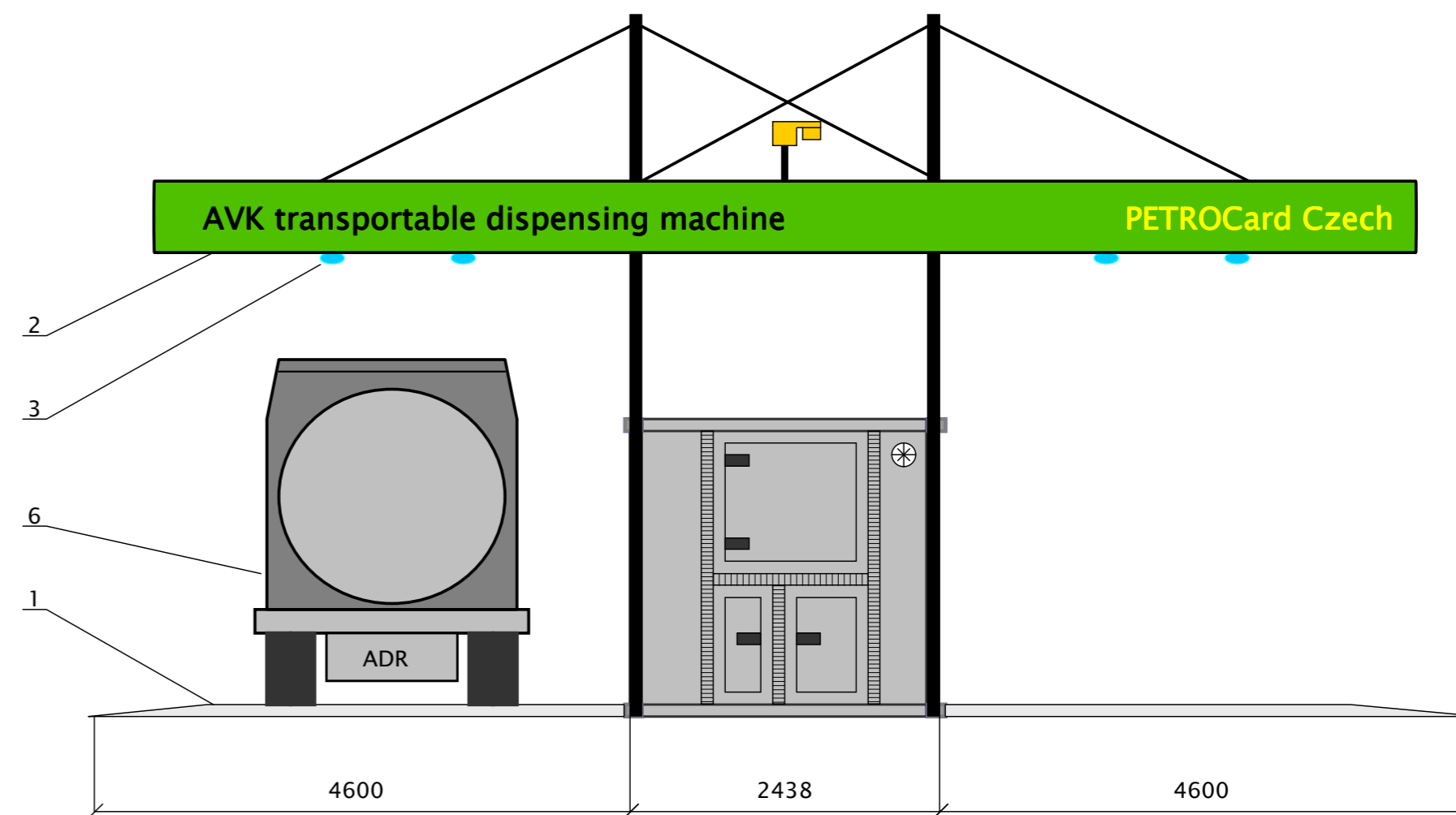
Čelní pohled
